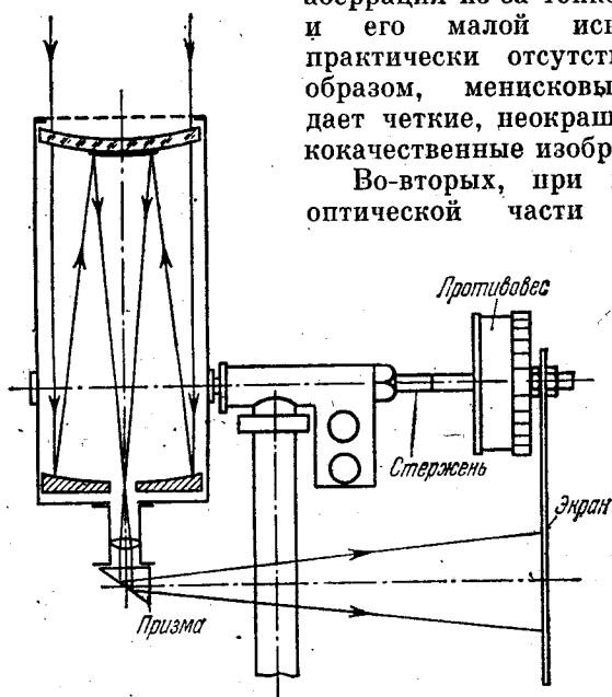
Рис. 16. Схема школьного менискового телескопа.
