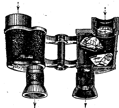
Рис. 12. Призмённый бинокль.
