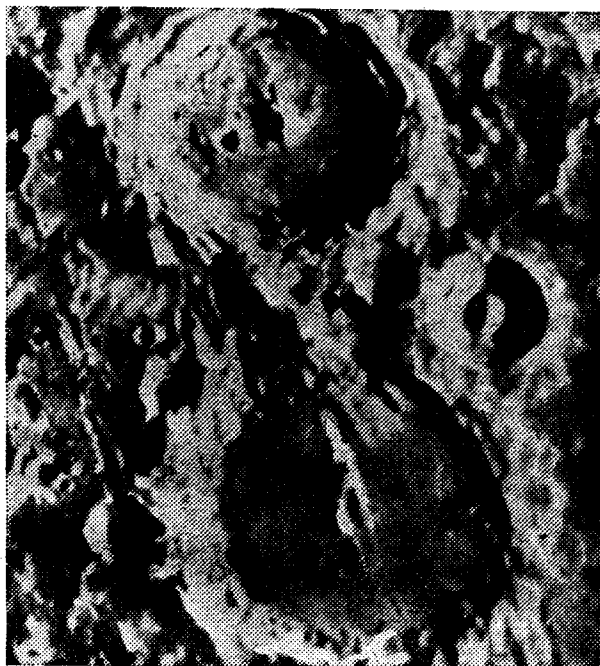
Рис. 95. Кратеры Альфонс (внизу), Арзахель (вверху) и Альбистрагий (справа).
