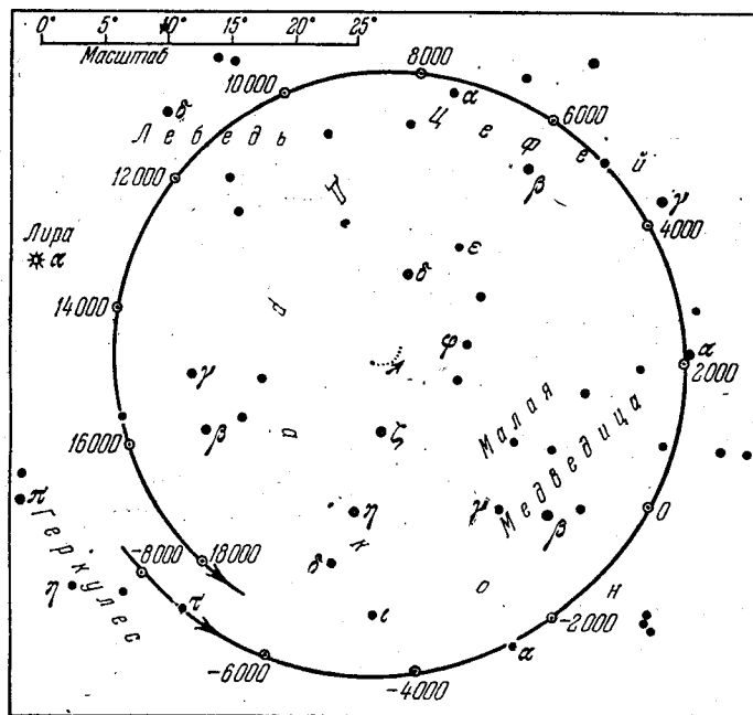
Рис. 29. Прецессионное перемещение полюса мира по созвездиям.
