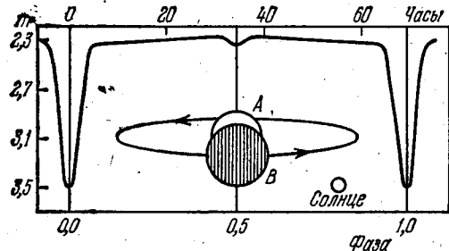
Рис. 41. Схема изменения блеска Алголя.
