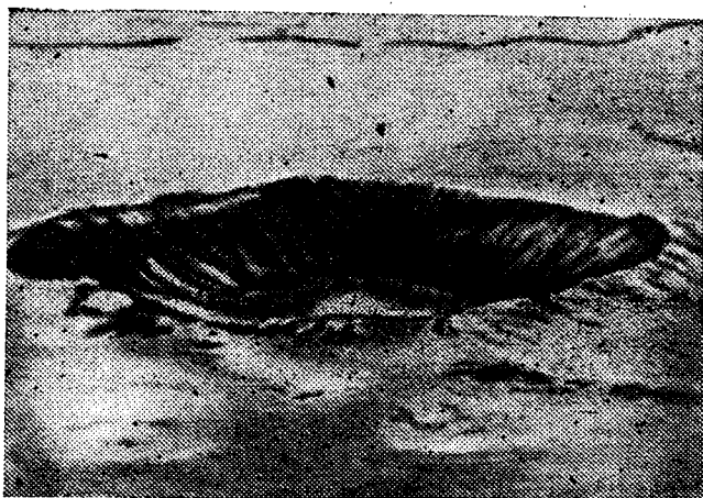
Рис. 83. Аризонский метеоритный кратер.
