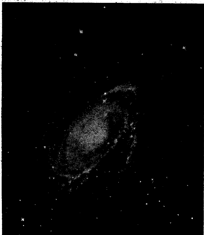
Рис. 34. Галактика М 81.
