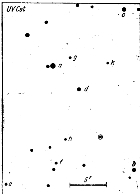
Рис. 47. Окрестности звезды UV Кита.
