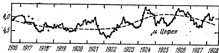
Рис. 37. Кривая блеска \mu Цефея.
