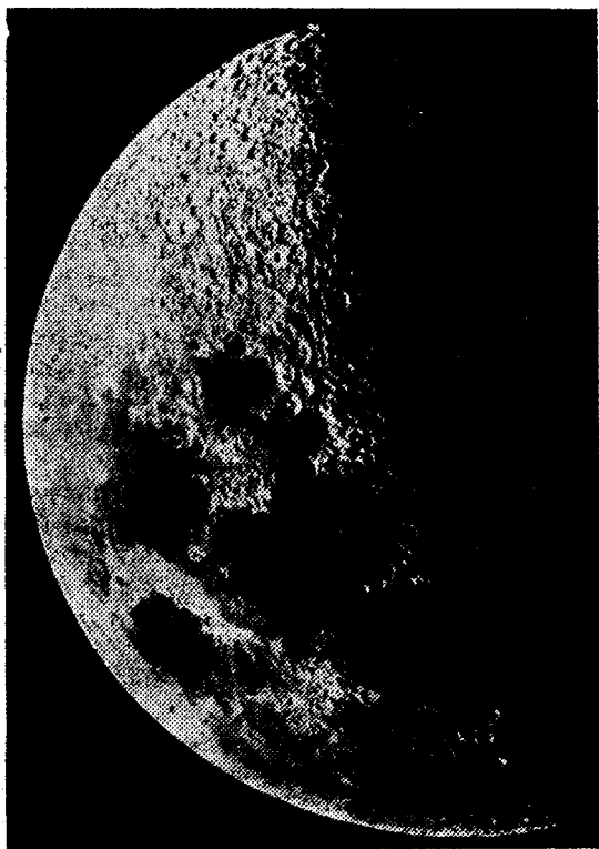
Рис. 88. Луна в фазе первой четверти (изображение перевернутое).
