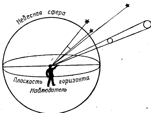
Рис. 19. Небесная сфера.
