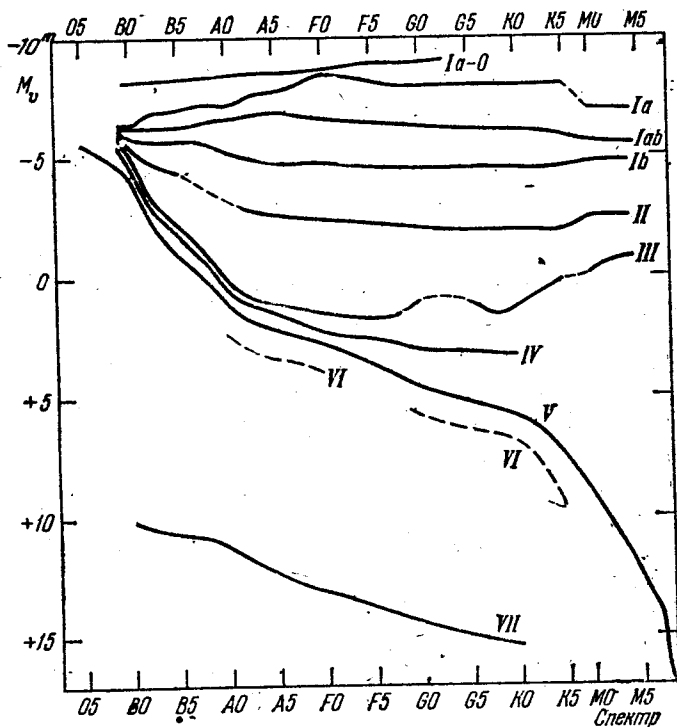
Рис. 3. Диаграмма Герцшпрунга — Рассела. Последовательности: Ia-0 — ярчайших сверхгигантов, Ia — ярких сверхгигантов, Iab — средних сверхгигантов, Ib — слабых сверхгигантов, II — ярких гигантов, III — слабых гигантов, IV — субгигантов, V — главная последовательность, VI — субкарликов, VII — белых карликов.
