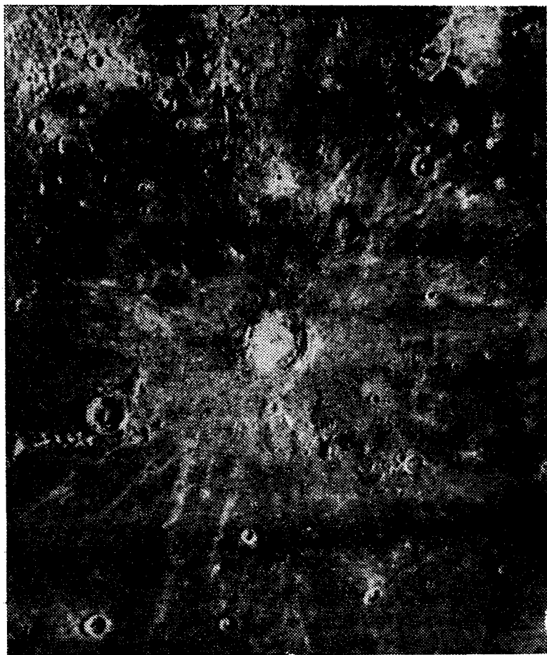
Рис. 93. Система светлых лучей кратера Коперник.
