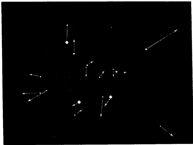
Рис. 43. Звездная ассоциация Персей II.
