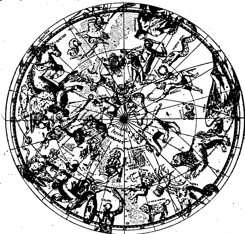
Рис. 1. Фигуры созвездий околополярной области в старинном звездном атласе.
