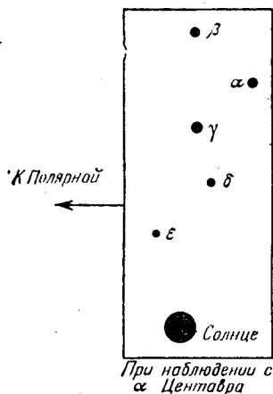
Рис. 73. Вид Солнца с α Центавра.
