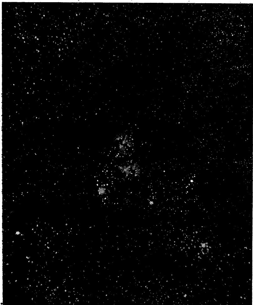
Рис. 69. Тройная туманность в созвездии Стрельца.
