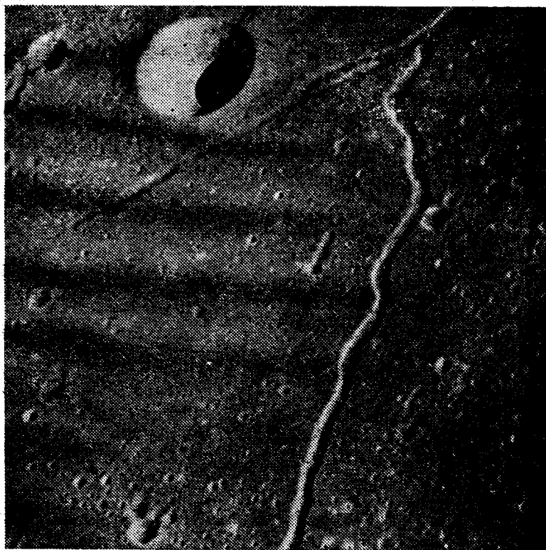
Рис. 105. Трещина Гигин (вверху) на видимом полушарии Луны и одна из лунных борозд (внизу), сфотографированная на обратной стороне Луны.
