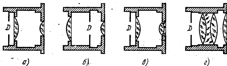
Рис. 15. Различные типы окуляров: а) Рамсдена, б) Гюйгенса, в) Кельнера (ахроматический), г) Аббе (ортоскопический).
