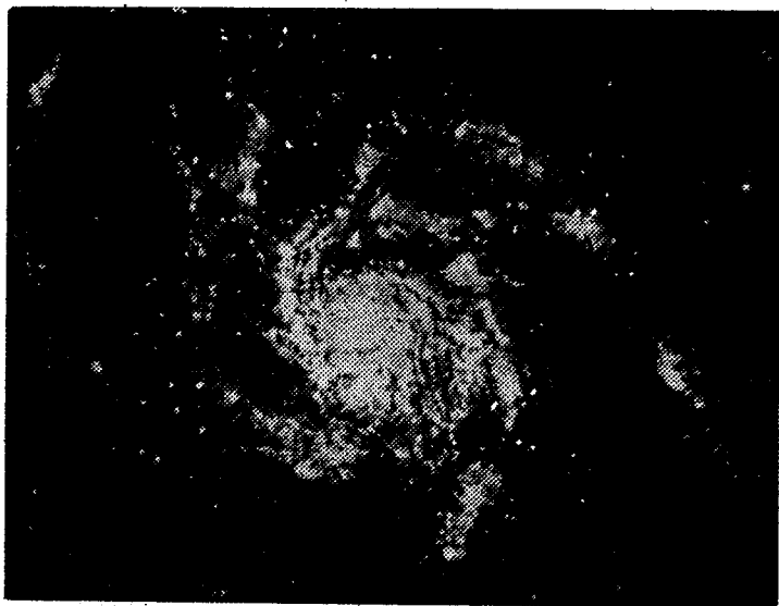
Рис. 33. Галактика М 101.
