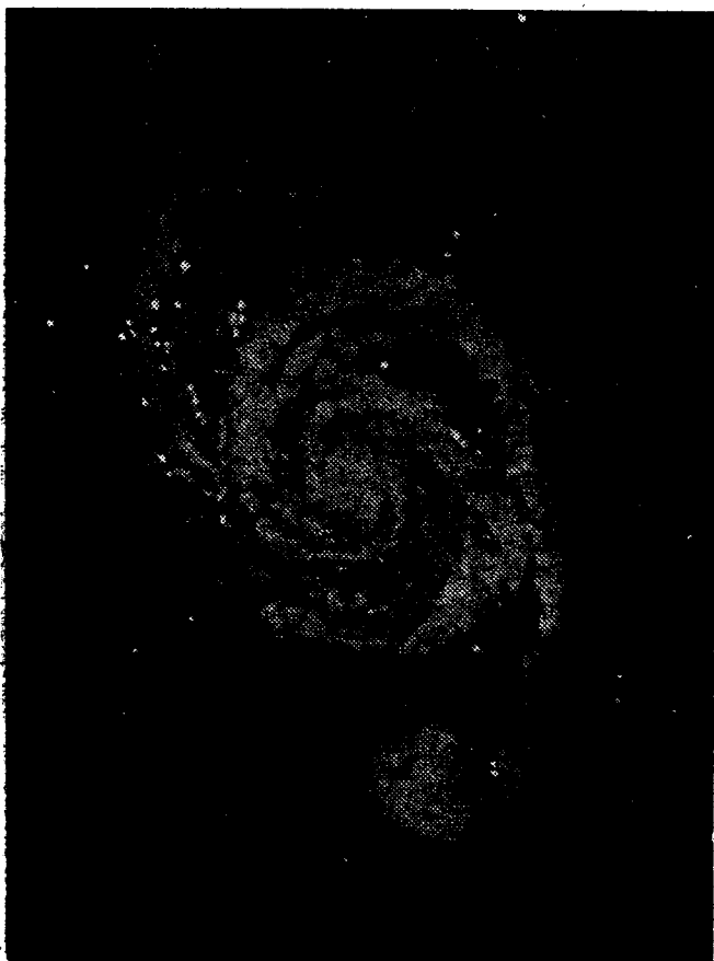
Рис. 5. Галактика М 51 из созвездия Гончих Псов.
