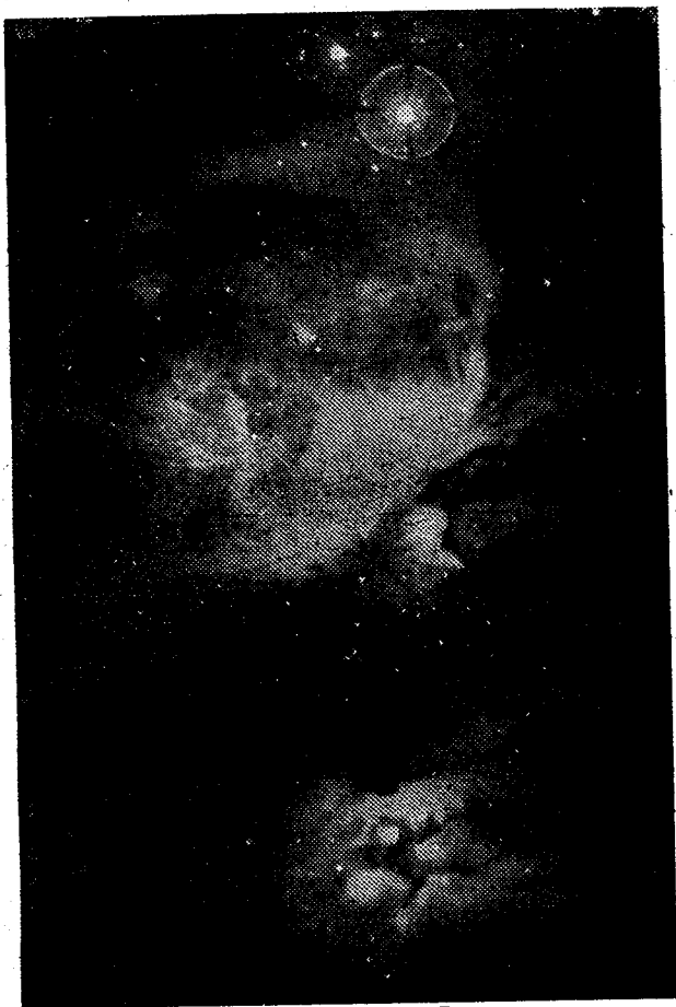
Рис. 49. Туманность Ориона.
