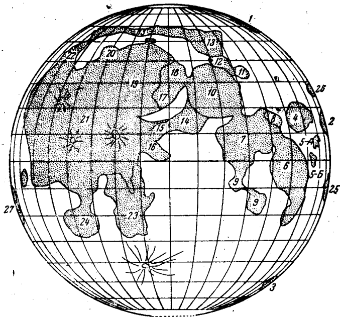
Рис. 78. Карта морей Луны (изображение прямое)..
