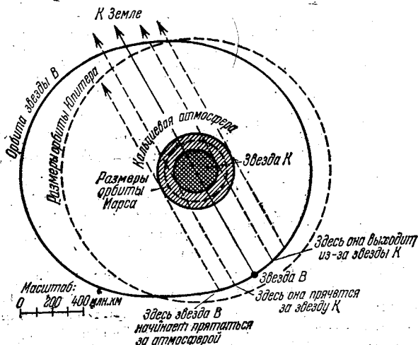
Рис. 55. Звезда \zeta Возничего.
