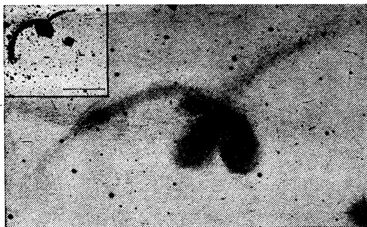
Рис. 8. Необычные галактики VV 79 (вверху слева), VV 243 — «Оса» (вверху справа) и VV 245 (внизу).
