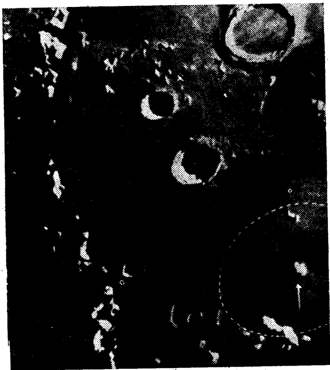
Рис. 91. Гора Питон (отмечена стрелкой). Штриховой линией помечен горизонт для наблюдателя, находящегося на вершине этой горы.
