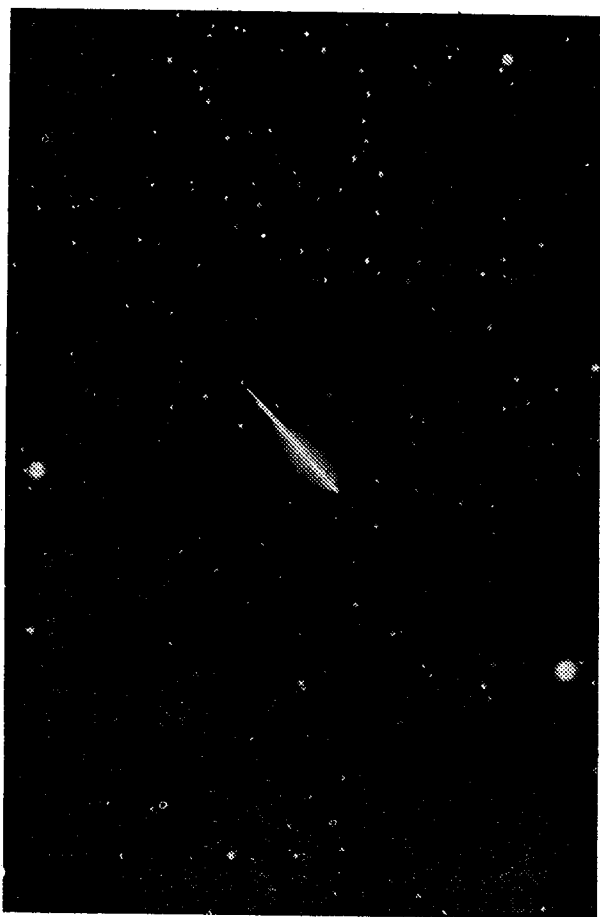
Рис. 75. Болид.
