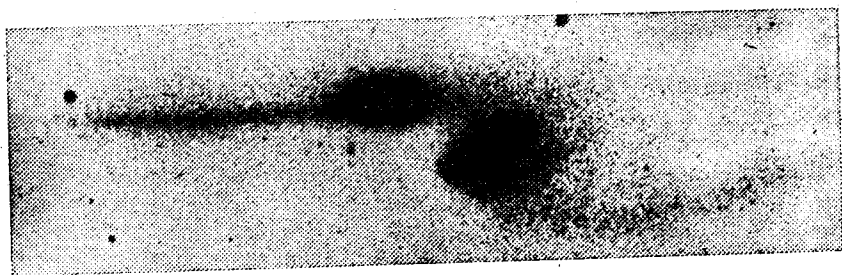
Рис. 7. Взаимодействующие галактики «Мышки».
