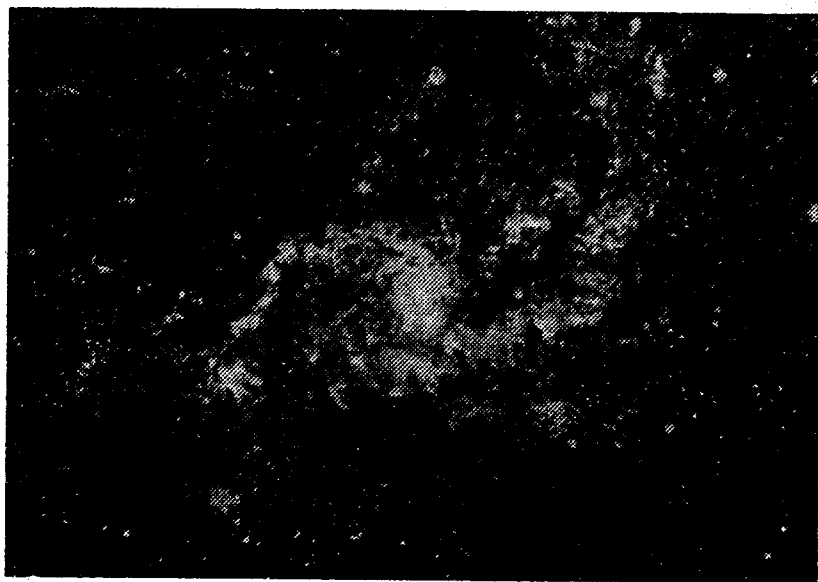
Рис. 45. Фотография галактики М 33.
