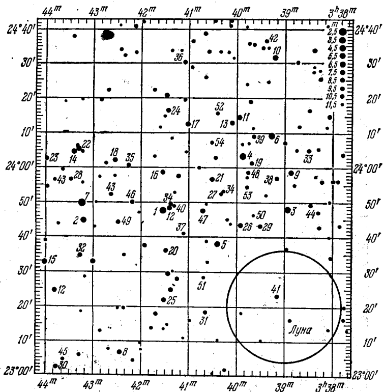
Рис. 50. Вид Плеяд в телескоп (кружком обозначены размеры лунного диска): 1 — Альциона, 2 — Атлас, 3 — Электра, 4 — Майя, 5 — Меропа, 6 — Тайгета, 7 — Плейона, 9 — Целена, 11 — Астеропа.
